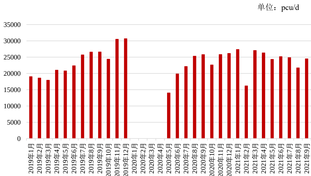
图：嘉通高速 2019-2021 年 1-9 月逐月标准车流量情况
